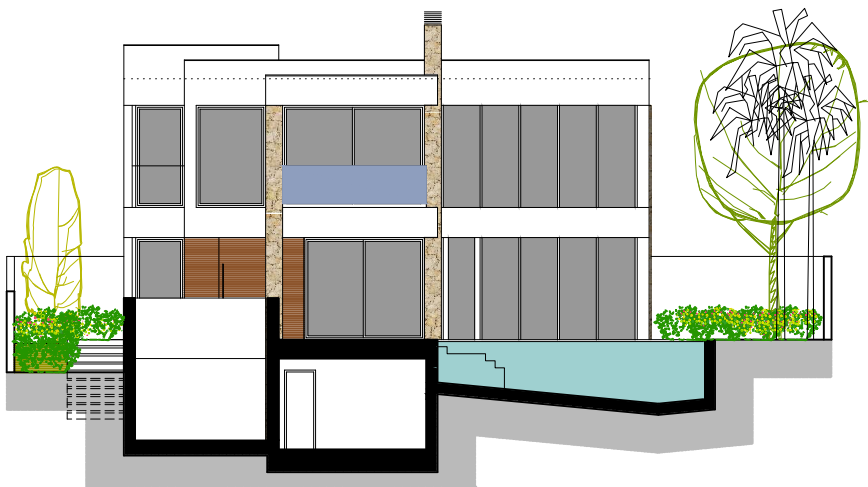
ALZADO OESTE FACADE WEST
