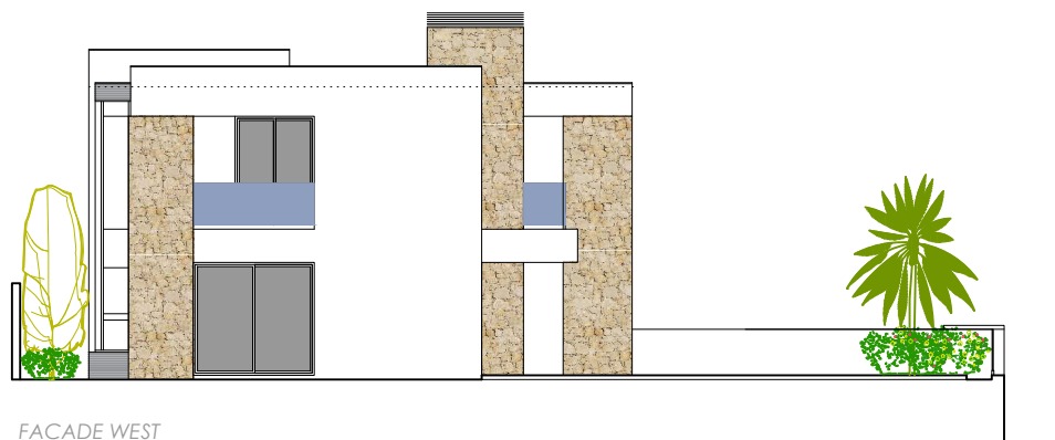
ALZADO OESTE FACADE WEST
